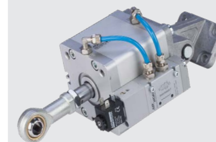
Solution spéciale - Vérin compact ISO 21287 Solución especial - Cilindro compacto ISO 21287
